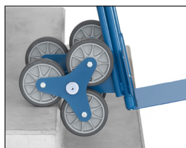
Roues en étoile à 3 branches TK1325 | TK1326
