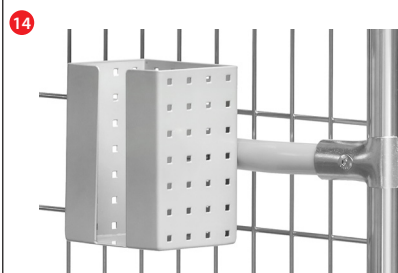
Porte-lecteur
