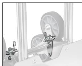
Blocage des roues en étoile 1770 Option pour les diabes escaliers AK1325 et AK1326.
